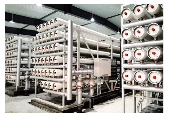
补连塔区域矿井水处理厂反渗透膜浓缩过滤。
